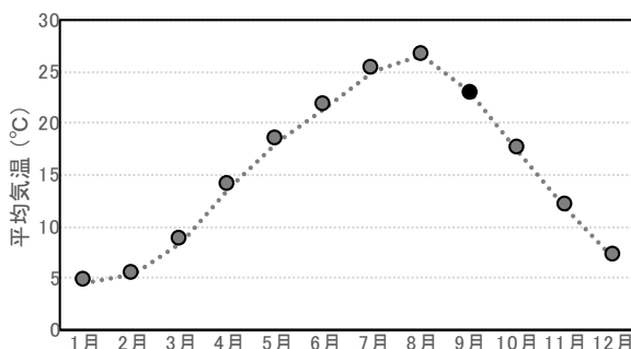
図1 海老名市における過去30年間の平均気温
