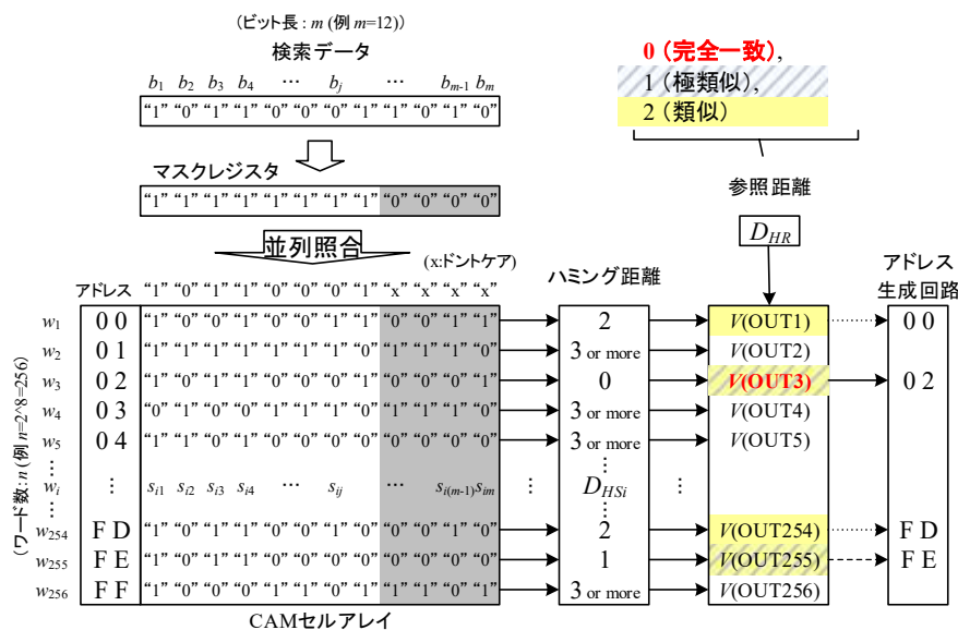
図1: ハミング距離検索連想メモリのブロック図
